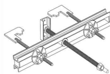
Réglette d'about réglable
